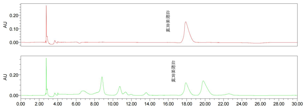
图 1 盐酸麻黄碱对照品及柏麻提取物色谱图
